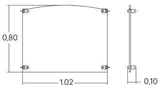
Szerelés G3425 oszlopokra
